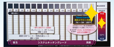
システムキッチン扉 材質比較
